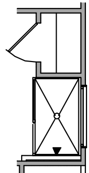
OPTIONAL SHOWER 5"
